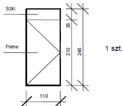
PARCHOCIN – WYKAZ STOLARKI DRZWIOWEJ (elew. wsch.)
